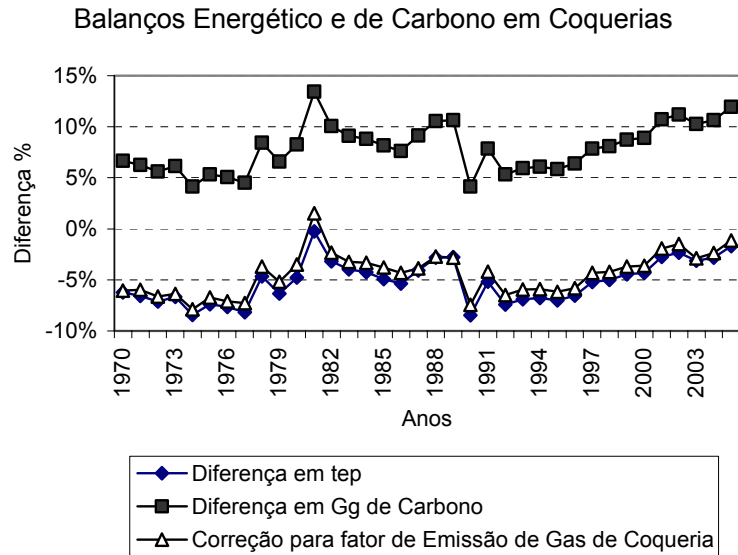
FIGURA 4.4: Balances de Energia e de Carbono em Coquerias mostrando os valores obtidos com os coeficientes 29,5 e 13,0 tC/TJ (correção) para o gás de coqueria; os valores corrigidos do balanço de carbono praticamente coincidem com os do energético.
