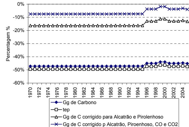
Figura 4.7 Balanços de energia e de carbono em carvoarias com correções (para massa de carbono) para os rejeitos e para as emissões.
