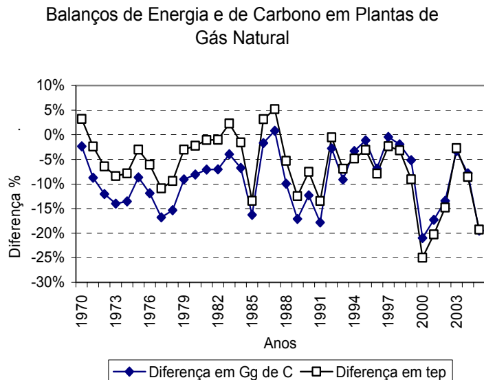
FIGURA 4.2: Balanços de Energia e de Carbono em Plantas de Gás Natural
