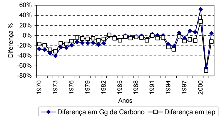
FIGURA 4.5: Balanços de Energia e de Carbono em Usinas de Gaseificação
